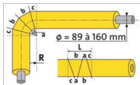
Coupe à 2 onglets.
