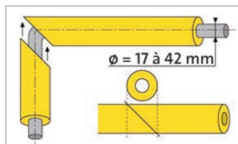
Coupe complète à 45°.
