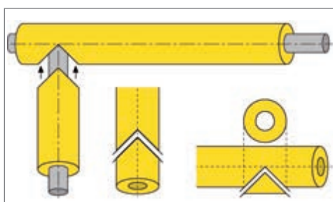
Coupe à 45° jusqu'à l'axe de la coquille.
