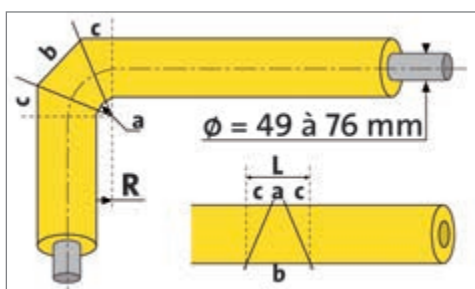
Coupe à 1 onglet.
